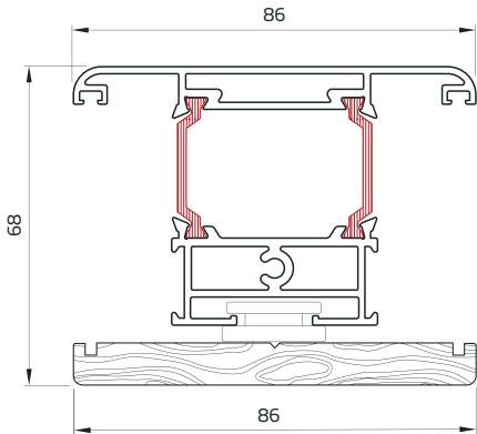
Traverso Montante
