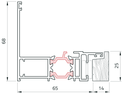
Telaio piano
