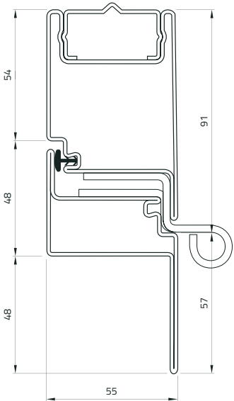
Nodo laterale
