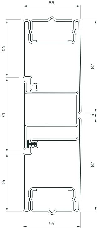
Nodo centrale
