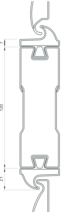
Nodo fascia
