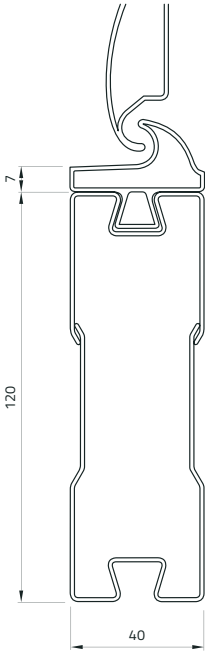
Nodo inferiore
