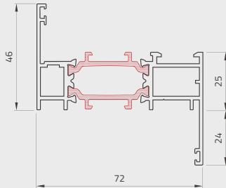
Telaio a ZETA 25 mm ZETA frame 25 mm
