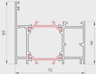
Telaio maggiorato Oversized frame
