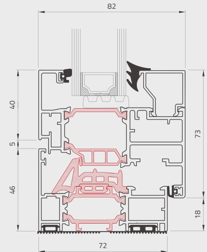
Sistema doppio vetro Double glass system
