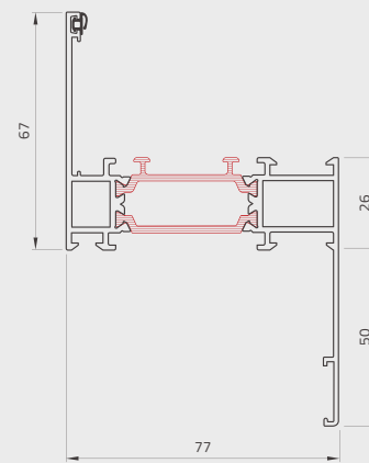
Telaio a ZETA 50 mm ZETA frame 50 mm
