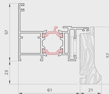
Telaio a ZETA 23 mm ZETA frame 23 mm
