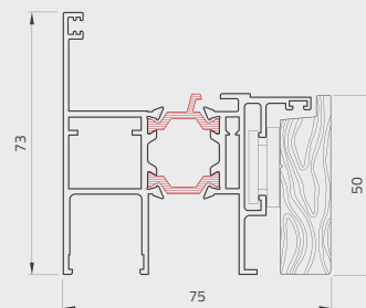
Telaio maggiorato Oversized frame
