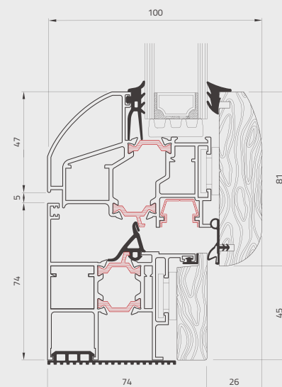
Sistema doppio vetro Double glass system
