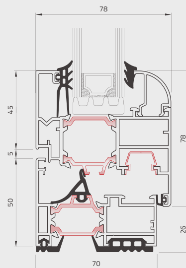
Sistema doppio vetro Double glass system
