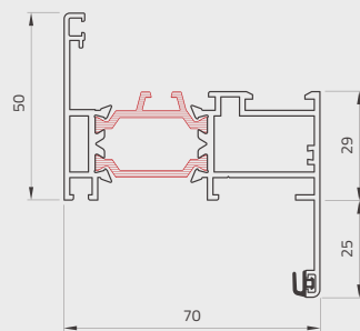
Telaio a ZETA 25 mm ZETA frame 25 mm
